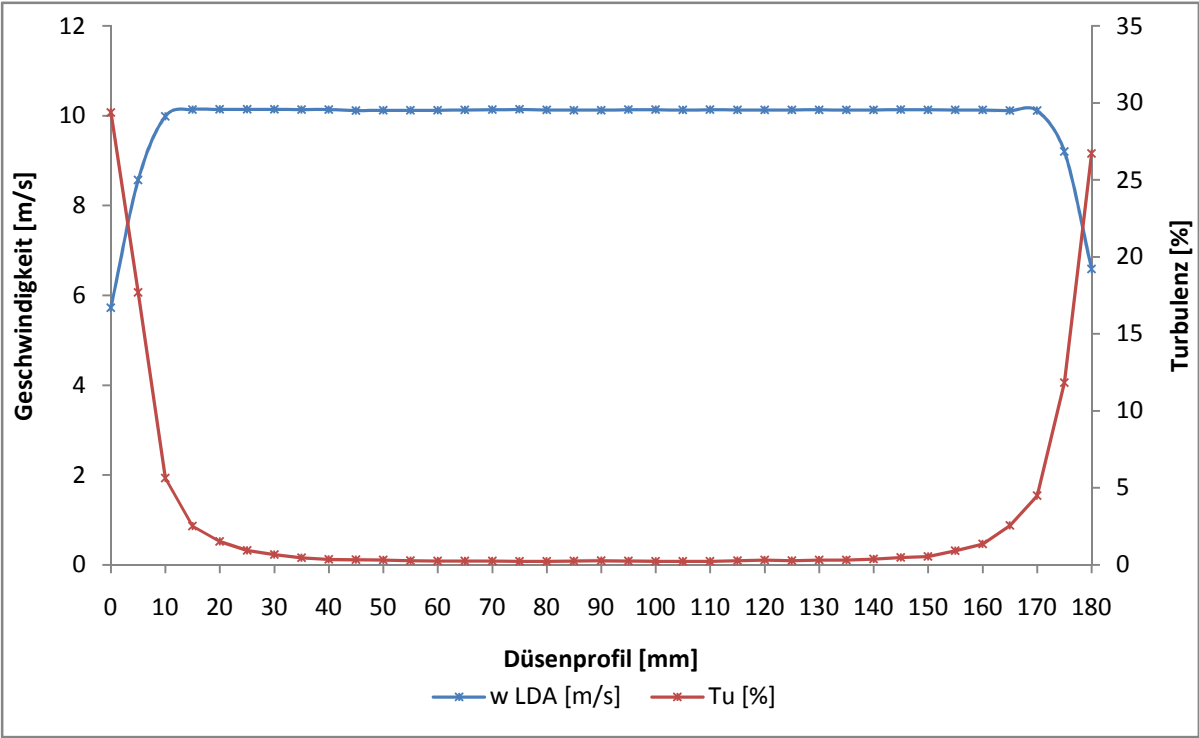
leerer Windkanal, 180 mm Düse, vertikal, 10 m/s
