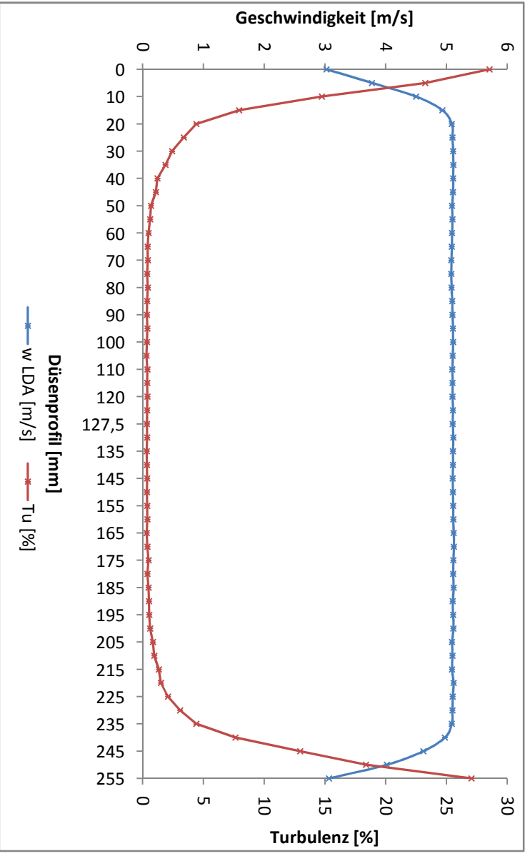
leerer Windkanal, 255 mm Düse, vertikal, 5 m/s
